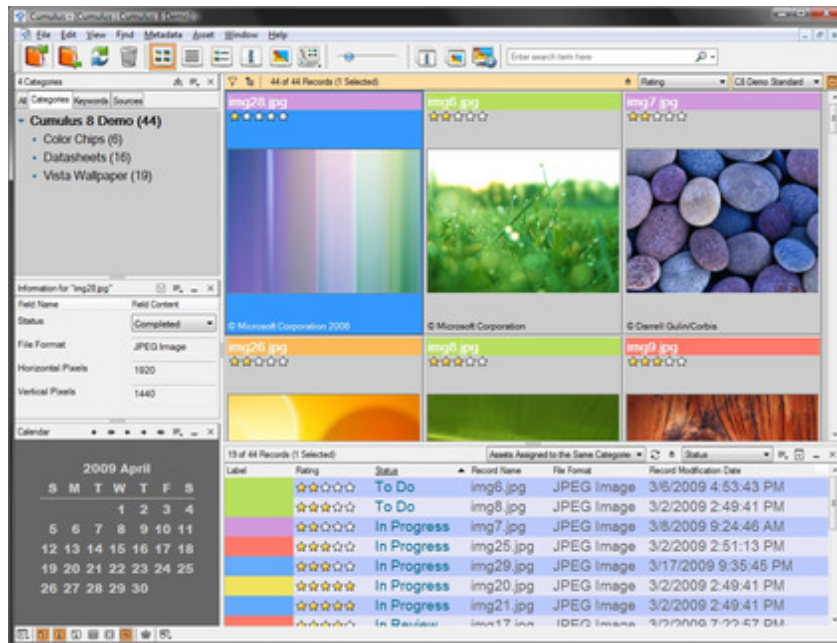
Cumulus 8 Benutzeroberfläche
